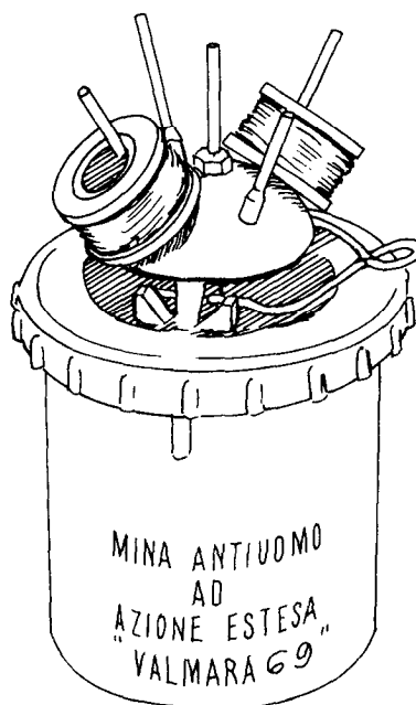
Valmara 69 antipersonnel mine (Italian)
